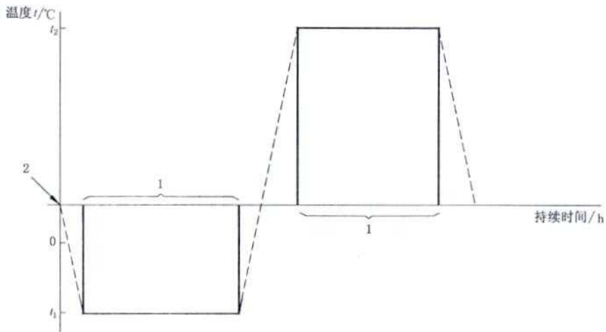
图 2 条件试验方法 15 的循环曲线：温度突变
